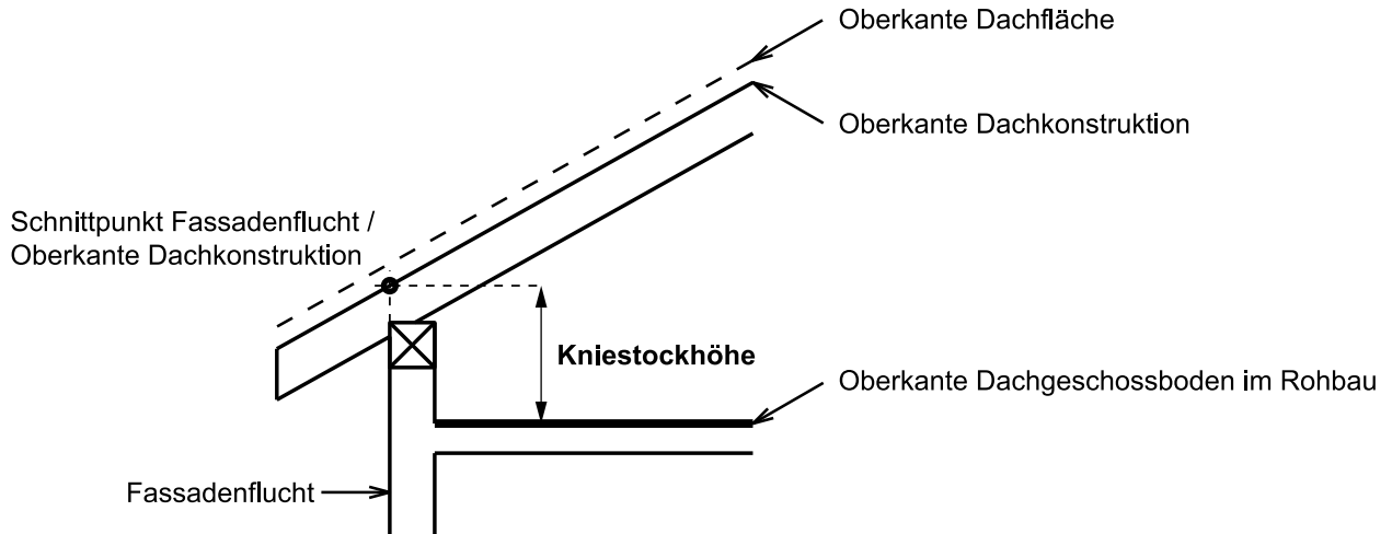
Figur 5.3 Kniestockhöhe
